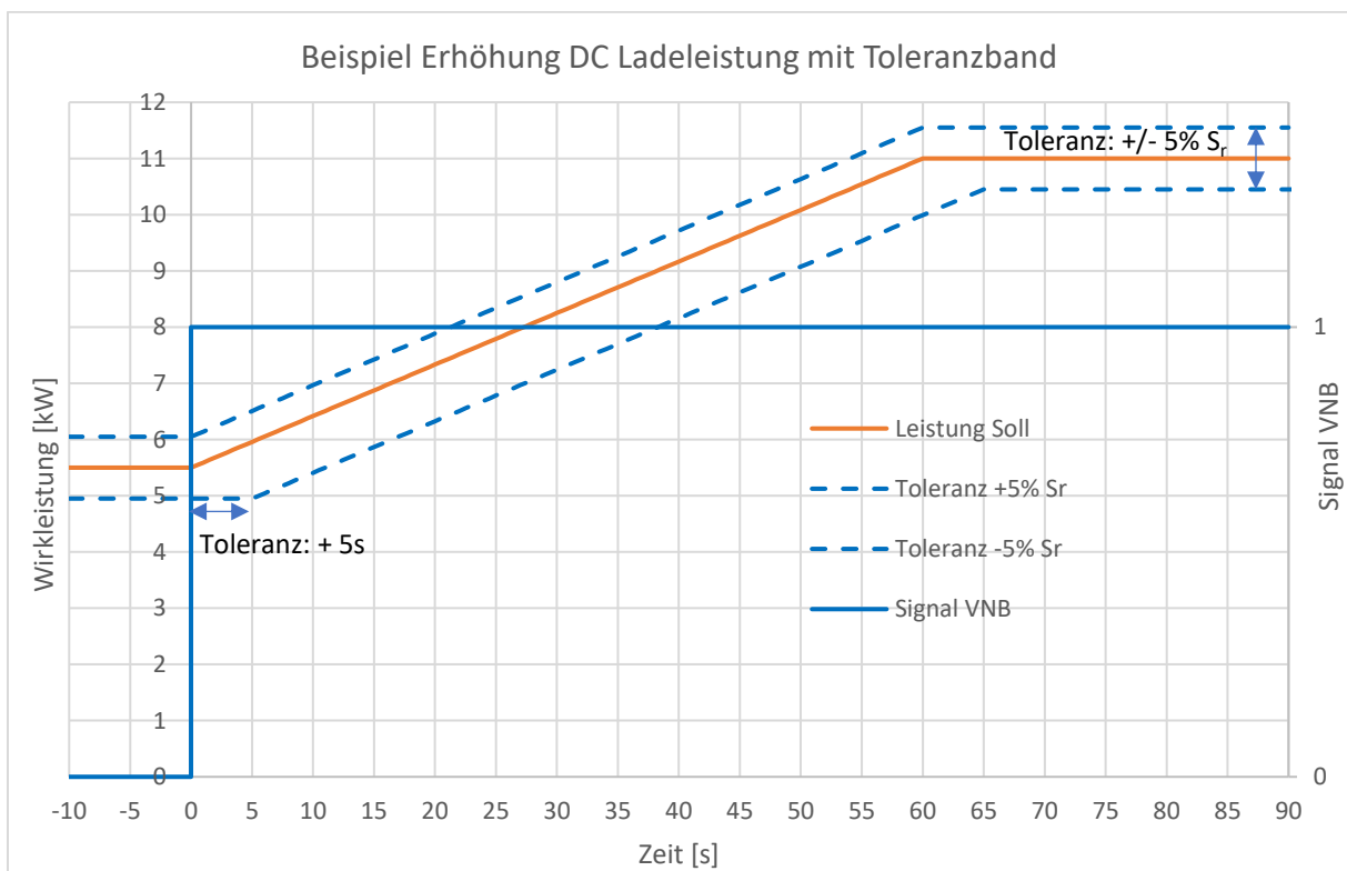
Diagramm 5 Toleranz DC-Ladestelle (Beispiel)
