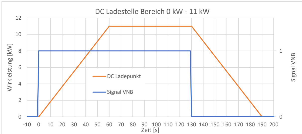
Diagramm 4 Verhalten DC-Ladestelle im Bereich zwischen 0 kW und 11 kW
